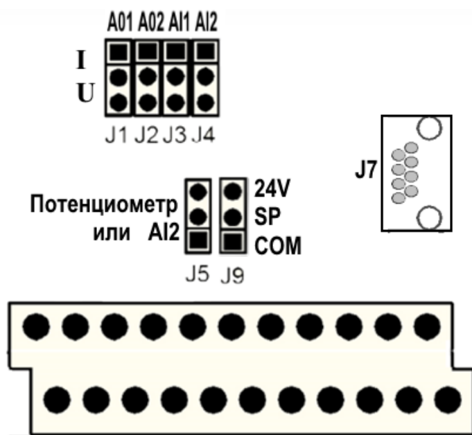
Рис. 2-8. Поле для установки перемычек
