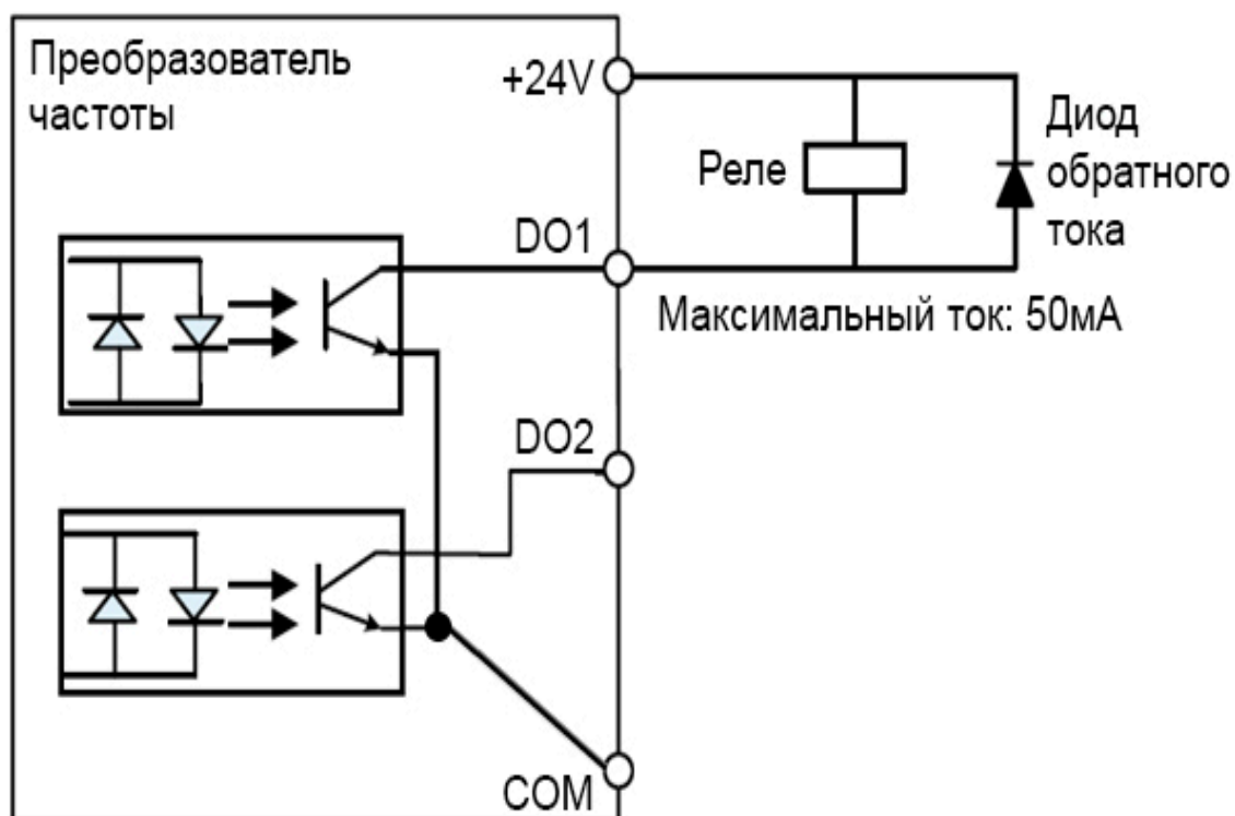
Рис. 2-7. Дискретный выход
