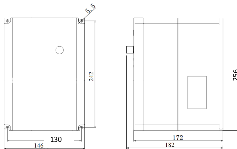
Рис. 1-5. Габаритные размеры преобразователей частоты с мощностью от 5.5 кВт до 11 кВт (380В) и 3.7 кВт (220В)
