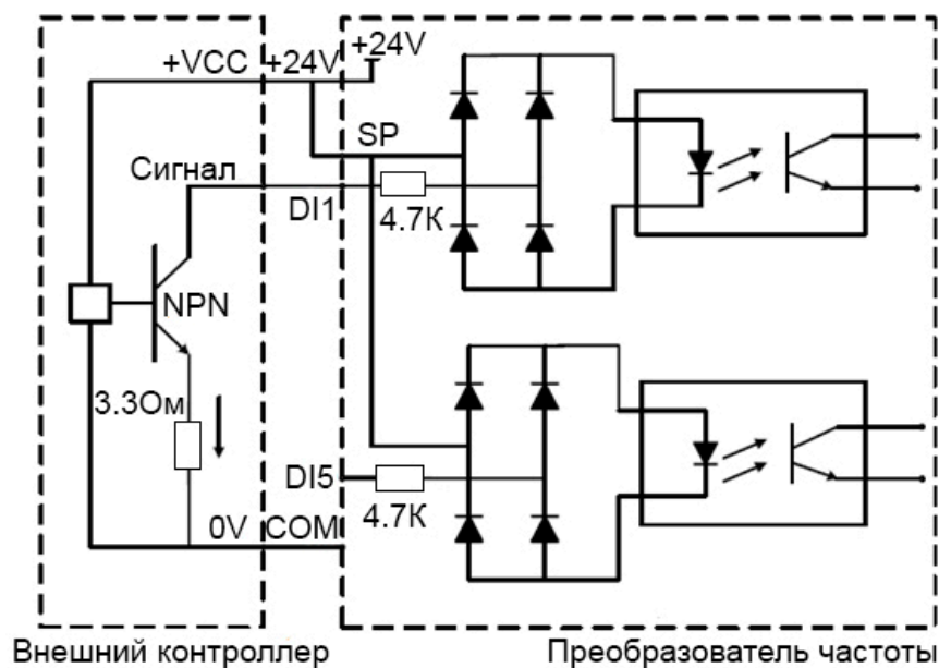
Рис. 2-5. NPN-вход
