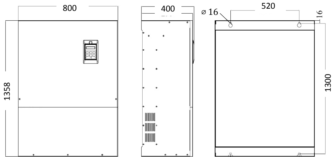
Рис. 1-14. Габаритные размеры преобразователей частоты с мощностью от 315 кВт до 400 кВт
