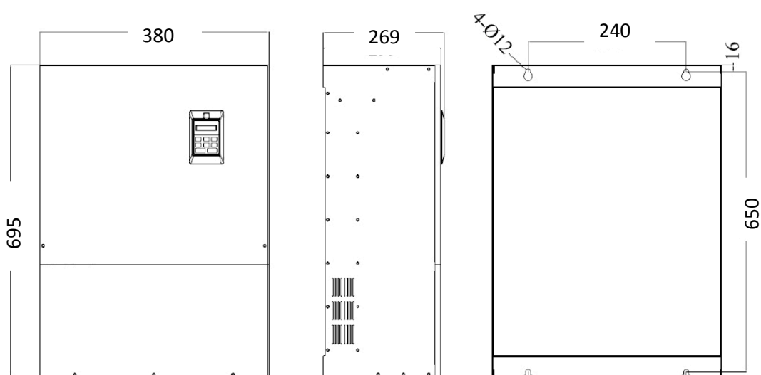
Рис. 1-9. Габаритные размеры преобразователей частоты с мощностью от 75 кВт до 90 кВт
