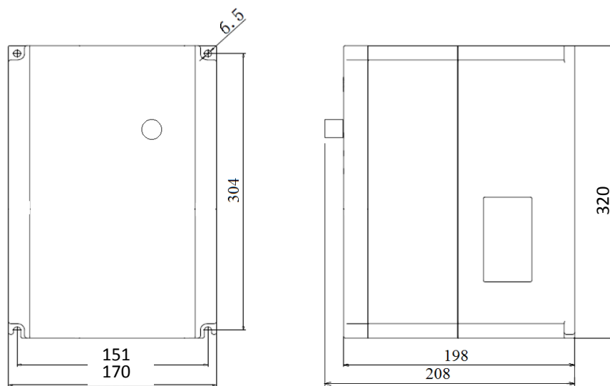
Рис. 1-6. Габаритные размеры преобразователей частоты с мощностью от 15 кВт до 22 кВт
