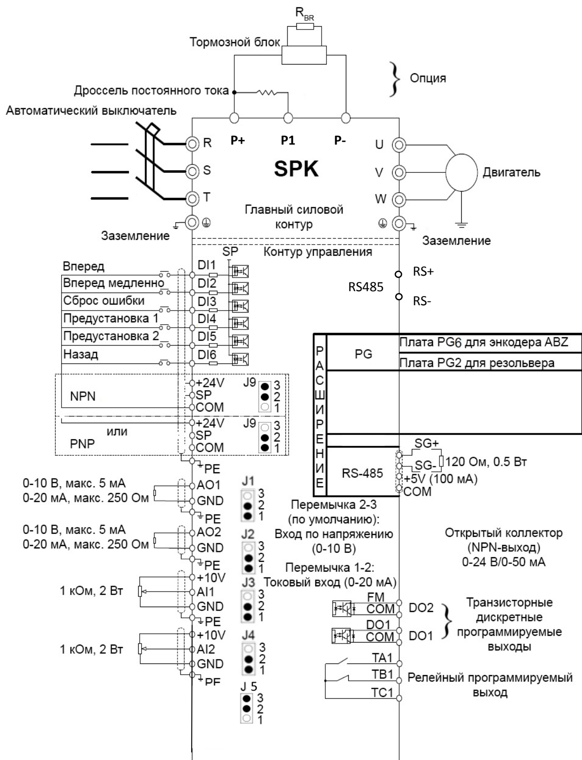
Рис. 2-2. Схема подключения преобразователя частоты с мощностью 45 кВт и более
