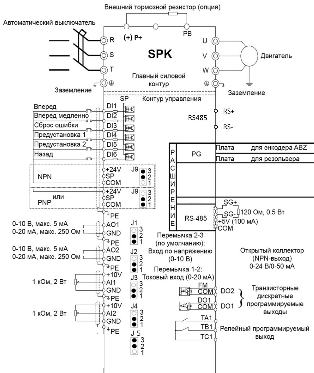
Рис. 2-1. Схема подключения преобразователя частоты с мощностью от 2.2 кВт до 37кВт.
