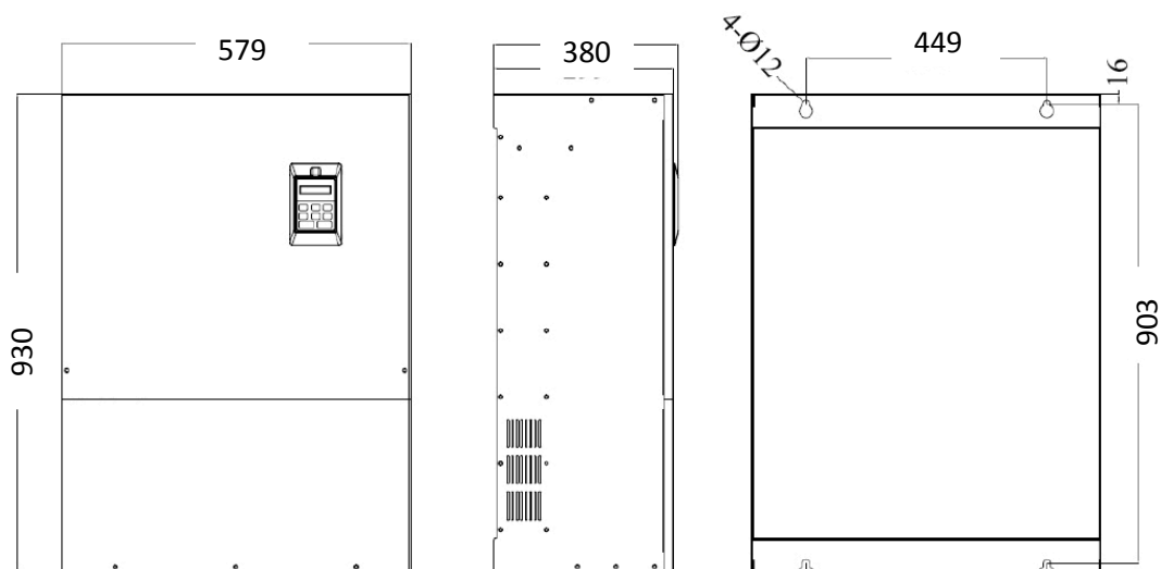
Рис. 1-11. Габаритные размеры преобразователей частоты с мощностью от 132 кВт до 160 кВт
