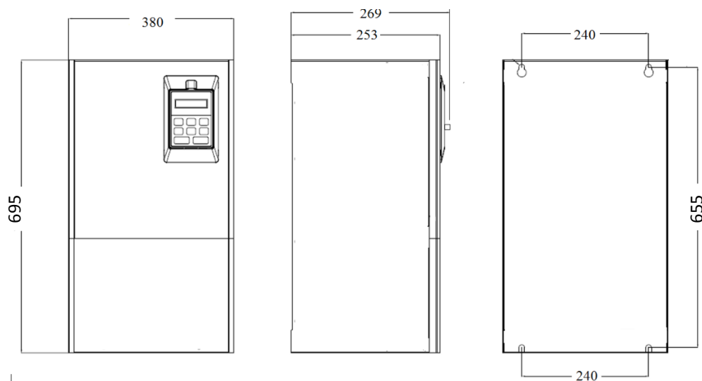
Рис. 1-9. Габаритные размеры преобразователей частоты с мощностью от 75 кВт до 90 кВт
