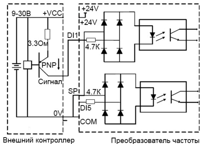
Рис. 2-6. PNP-вход
