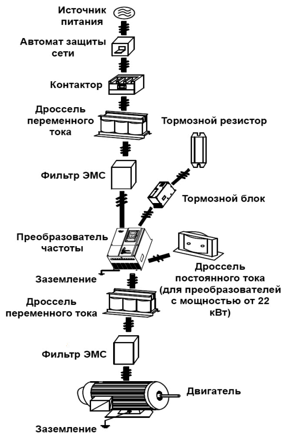
Рис. 1-2. Подключение преобразователя частоты
