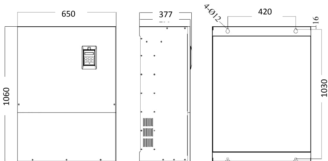
Рис. 1-12. Габаритные размеры преобразователей частоты с мощностью от 185 кВт до 200 кВт
