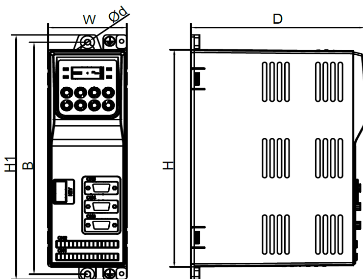
Габаритные размеры преобразователей частоты с мощностью от 0.4 кВт до 4.0 кВт (380В, тип G)
